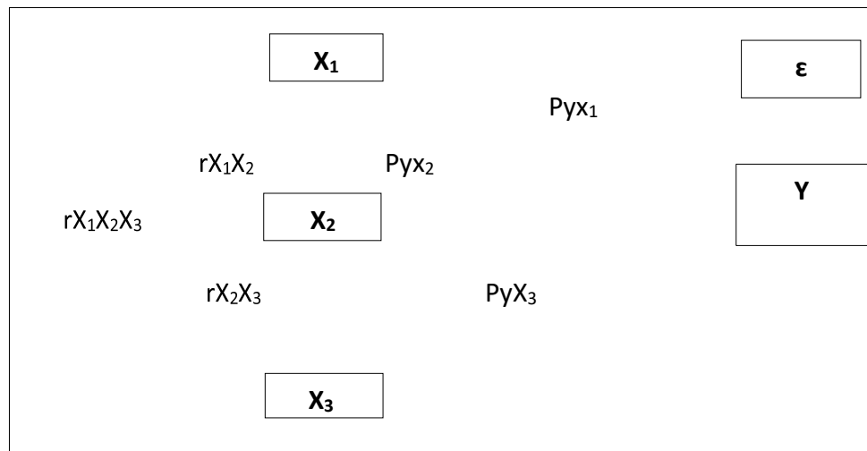
Gambar 1 Diagram Jalur Hubungan Kausal X_1, X_2, X_3 Terhadap Y
